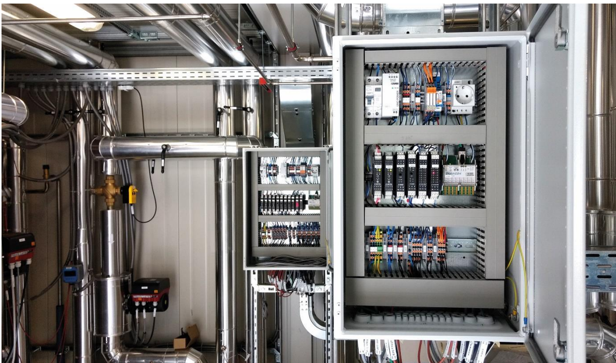
Bild 2: Schaltschrank mit Steuerungsmodulen
